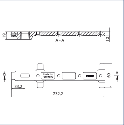
Опорная петля, модель CM
