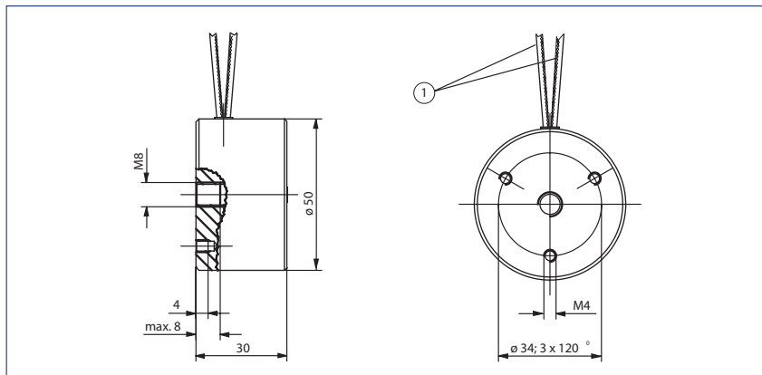
Контактный магнит, основная модель (оцинкованная катушка электромагнита без опорной пластины) для настенного монтажа или установки в любую конструкцию 1 = длина 200
