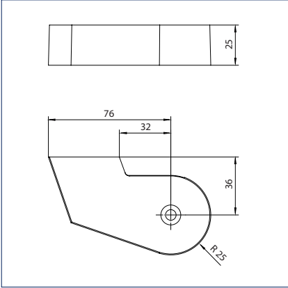
Крышки для опорных петель, модели DM, DB, EK, FK
