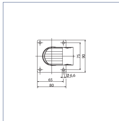
Цельнометаллический контактный магнит
