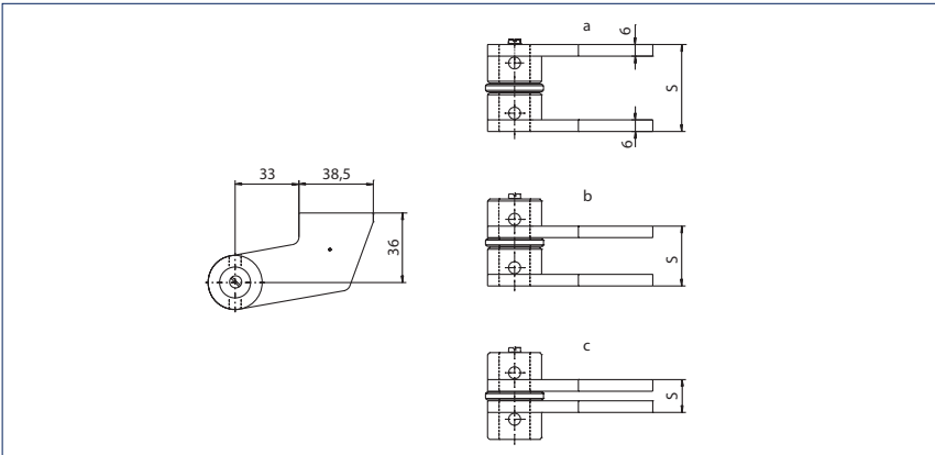
Подпятниковая петля, модель ЕК
