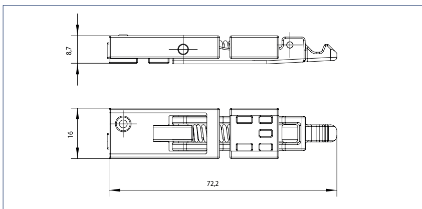
Механический фиксатор Boxer 12 мм
