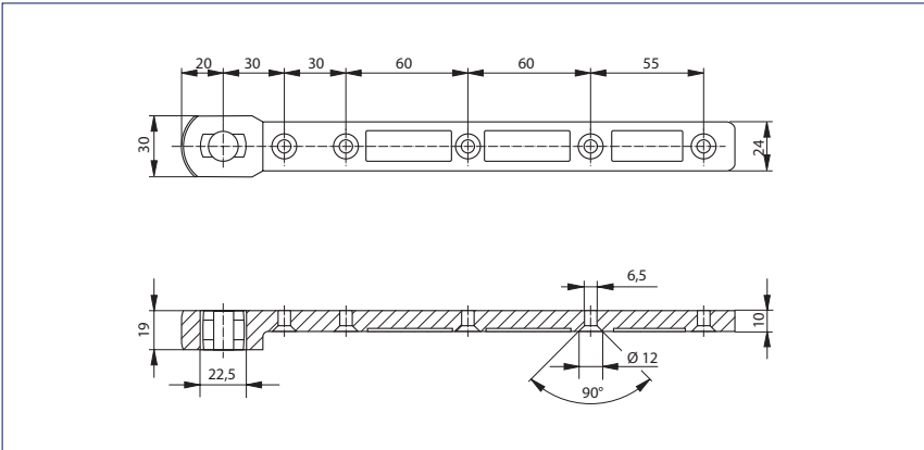
Опорная петля, модель S
