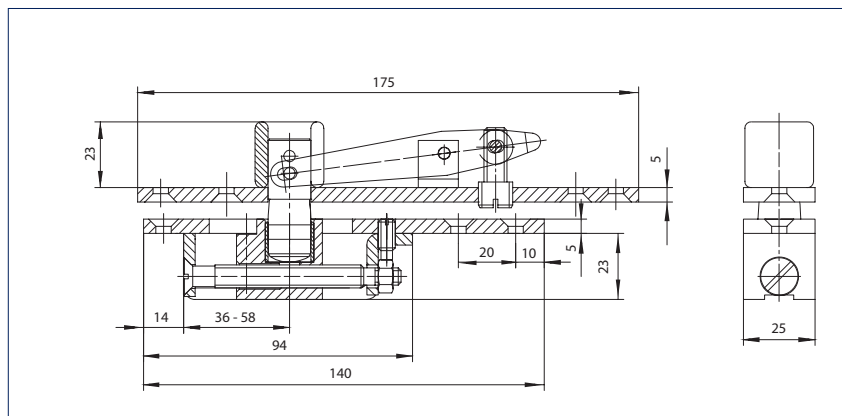
Регулируемая верхняя петля, модель С
