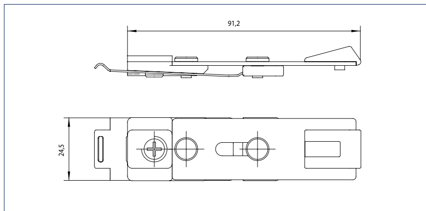
Механический фиксатор 20,7 мм скользящей шины Стандарт / T-Stop / Boxer
