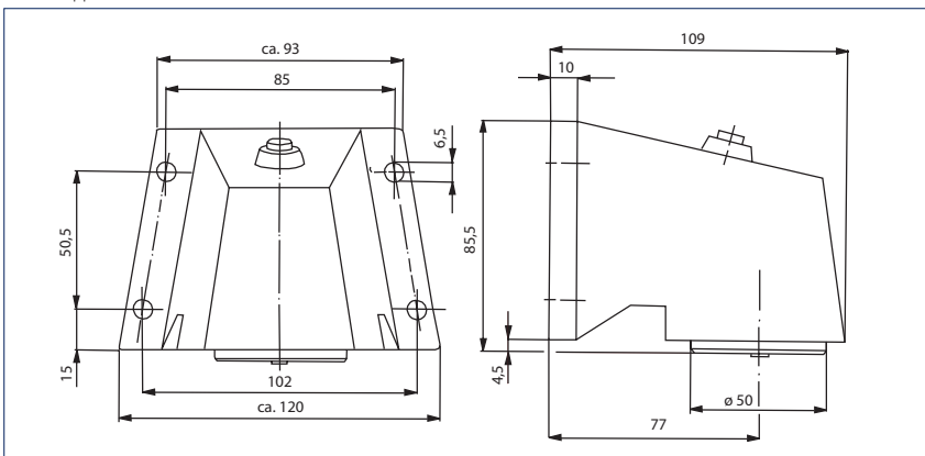
Контактный магнит, напольный монтаж, в алюминиевом корпусе с разъединяющей кнопкой
