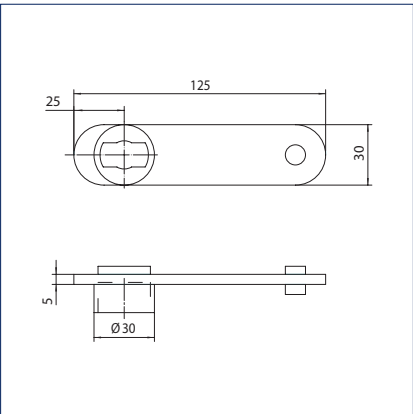
Опорная петля, модель S
