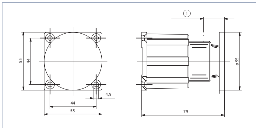
Ответная плата с пружинным амортизатором на монтажной плате с амортизирующей пружиной для мягкого пружинящего упора для тяжелых дверей
