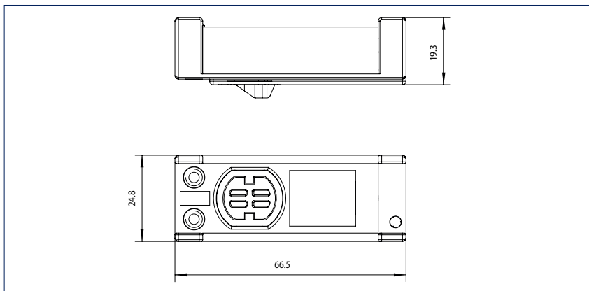
Механический фиксатор ISM
