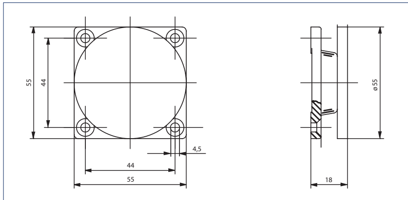
Ответная плата, стандарт, на монтажной плате с пружинной системой для адаптации под контактный магнит
