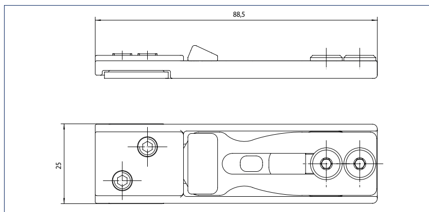
Механический фиксатор Ecline
