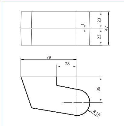
Крышки для подпятниковых дверей, модели DB, EK, FK
