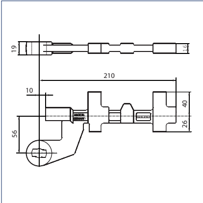
Опорная петля, модель DM
