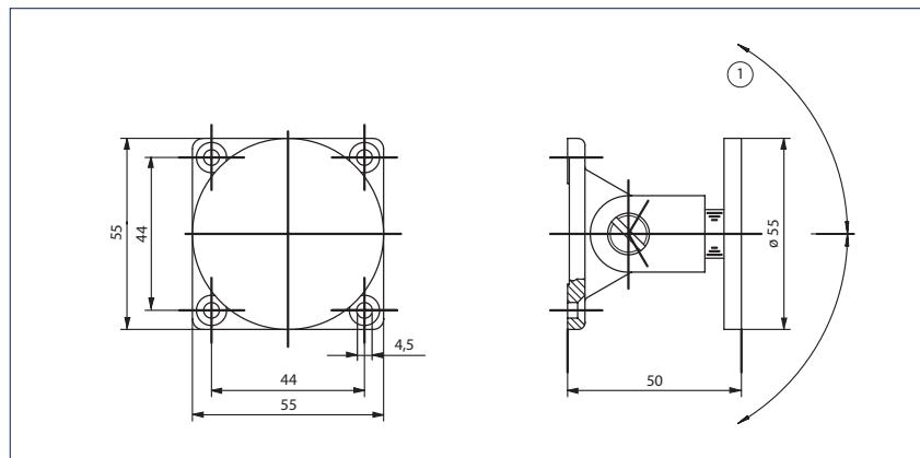
Ответная плата с шарниром на монтажной плате с дополнительной юстировкой для максимального углового положения между дверью и контактным магнитом
