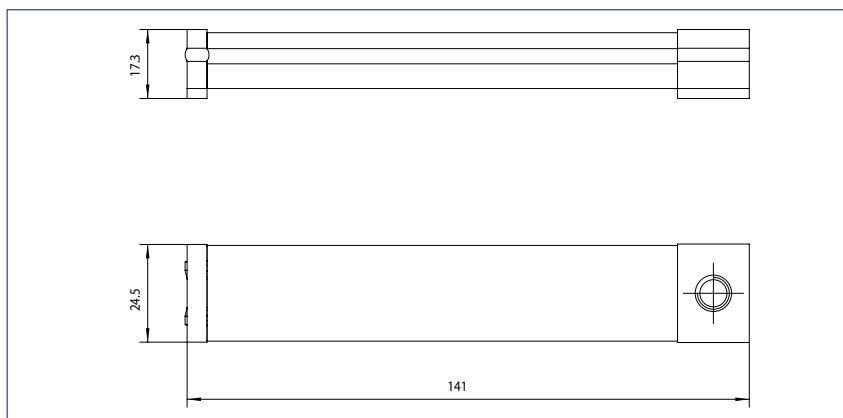
Упругий ограничитель открывания
