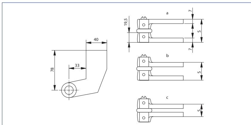
Подпятниковая петля, модель FK
