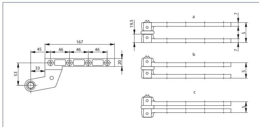
Подпятниковая петля, модель DB
