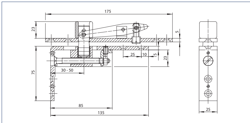
Регулируемая верхняя петля, модель В
