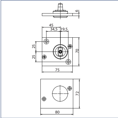
Вращающаяся опора с плоскоконической осью
