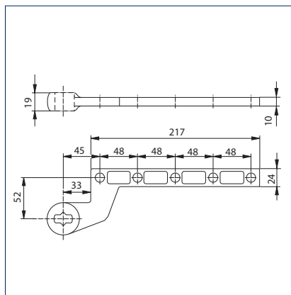
Опорная петля, модель DB
