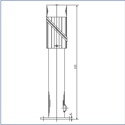
Цельнометаллический контактный магнит, L = 335 мм
