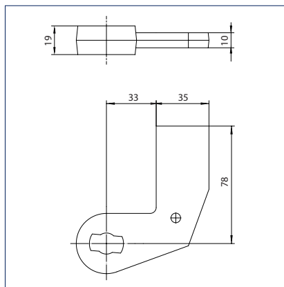
Опорная петля, модель FK
