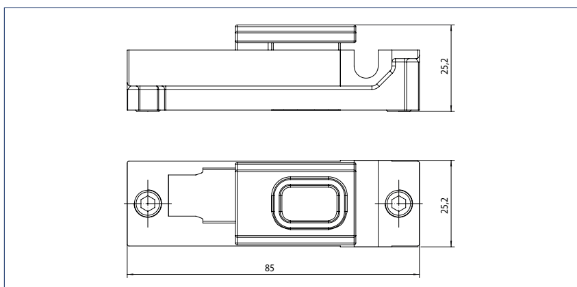
Упругий ограничитель открывания для скользящей шины E/R/ISM
