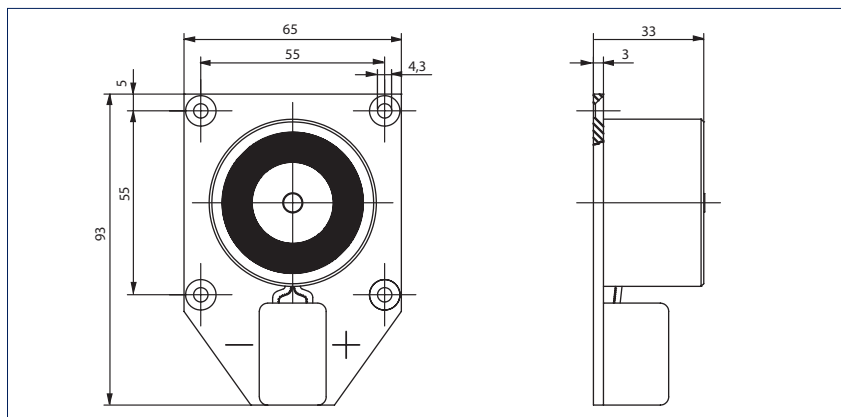
Контактный магнит, настенный монтаж, с опорной пластиной
