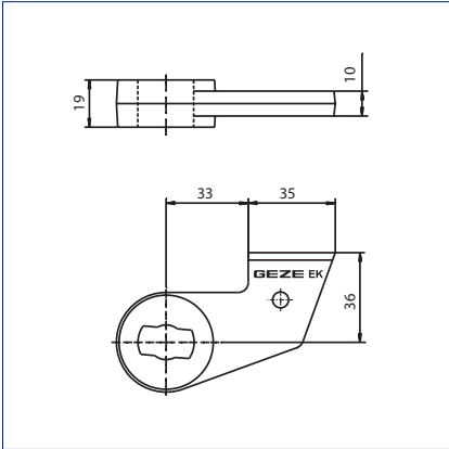
Опорная петля, модель ЕК
