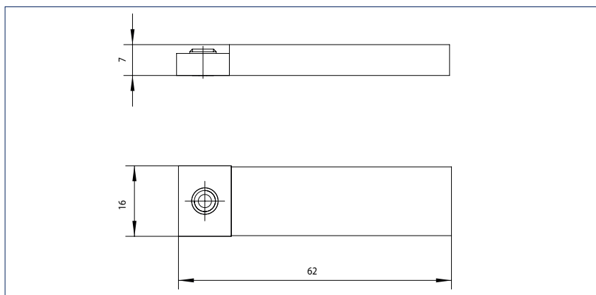
Ограничитель открывания 12 мм скользящей шины Boxer
